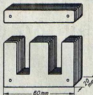
Rys.2 Orientacyjne rozmiary rdzenia transformatora
